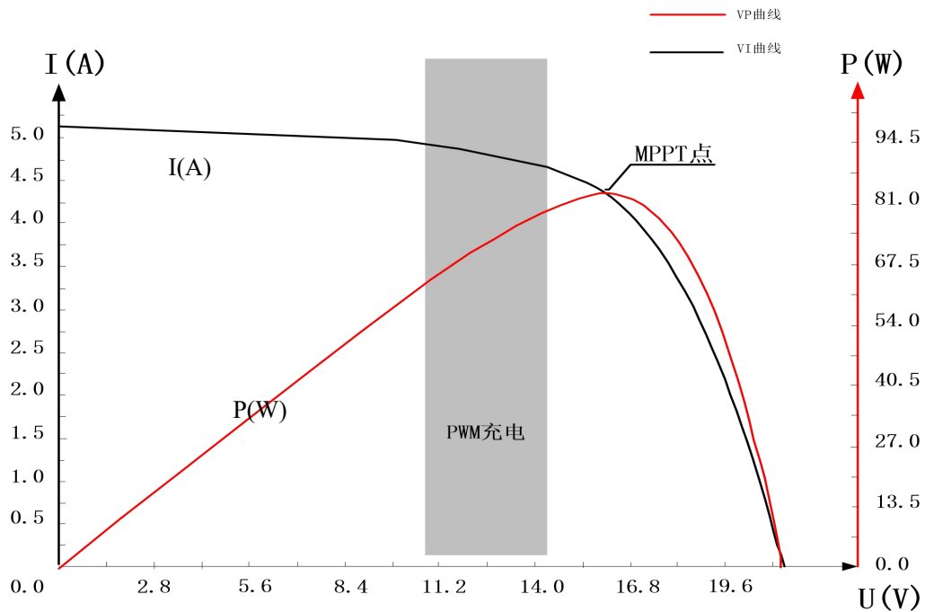
图 1-2 电池板输出特性曲线
