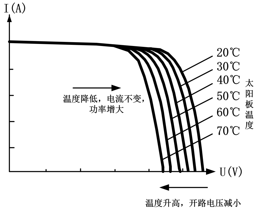
图 1-4 电池板输出特性与温度的关系
