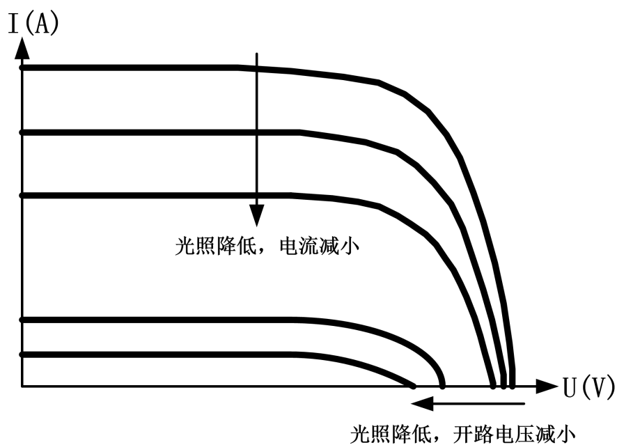
图 1-3 电池板输出特性与光照的关系
