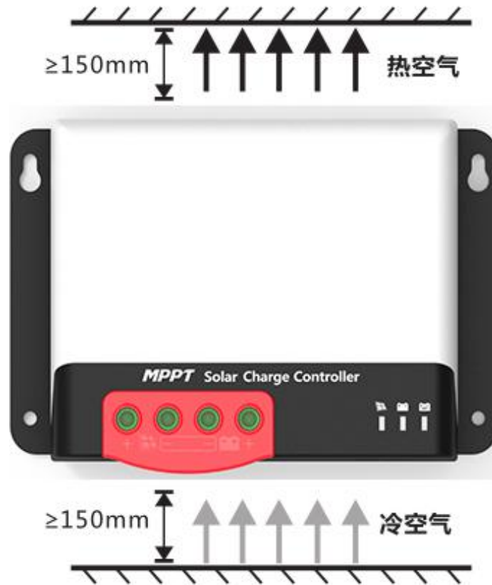
图2.1 安装和散热
